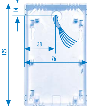
Bodenplatte des CO 2 -Fühlers
