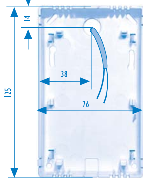
Bodenplatte des Fühlers
