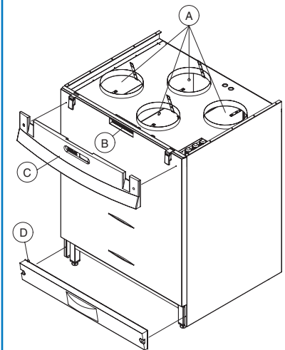
A Luftkanalschüsse B Messstutzen C Gerätepaneele D Sockelplatte
