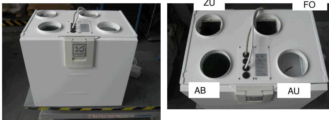
Bild 1: Prinzipbild des zentralen Lüftungsgerätes mit Wärmerückgewinnung vom Typ „VALLOPLUS 270 SE“ der Fa. VALLOX OY
