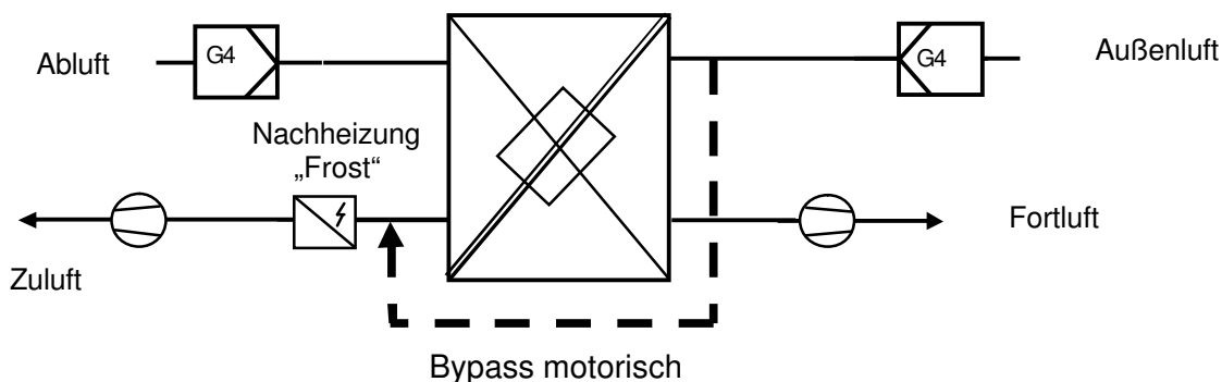
Bild 1: Prinzipbild des zentralen Lüftungsgerätes mit Wärmerückgewinnung vom Typ „VALLOPLUS 270 SE“ der Fa. VALLOX OY
