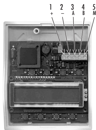
Reglereinheit von hinten
