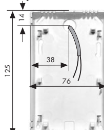
Bodenplatte des Fühlers
